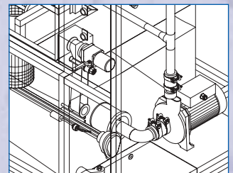
Bandölabscheider
