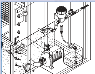
Waschmitteldosierung
