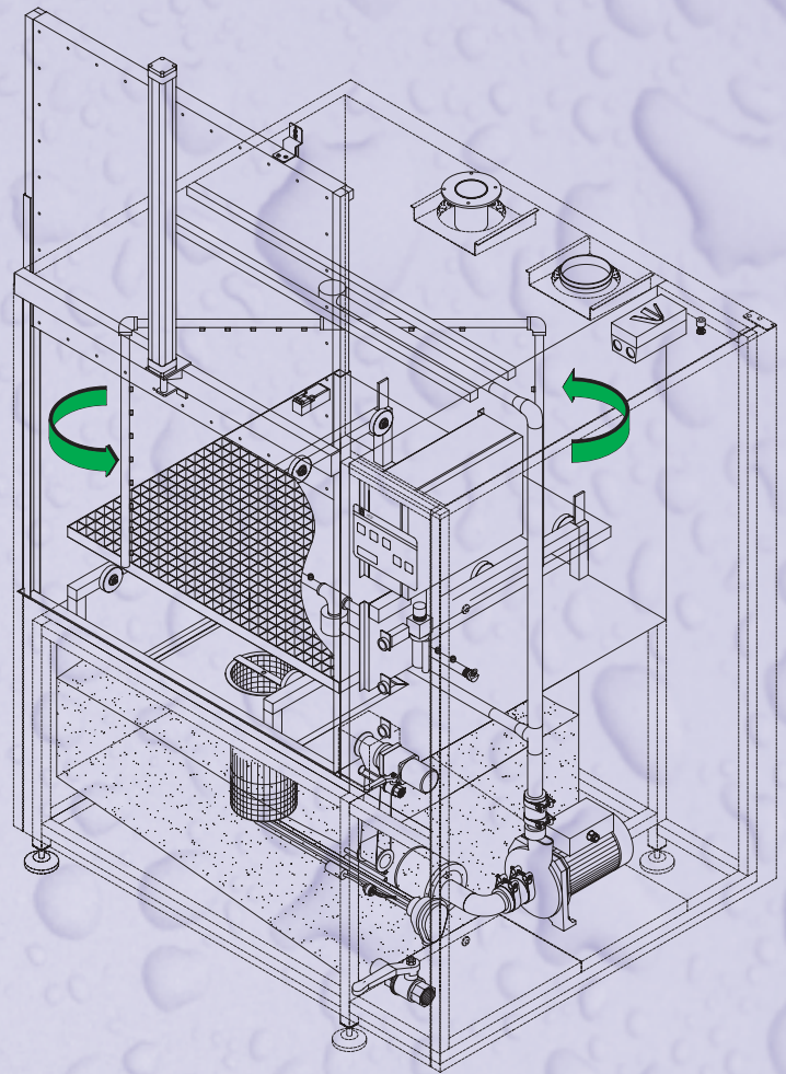
DF Standardmodell
