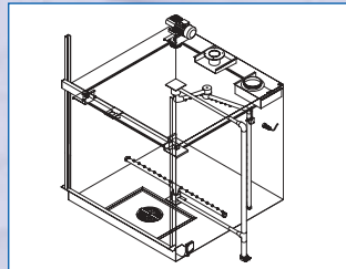
HEVISION Düsensystem
