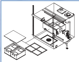
Waschkorbbeinrichtung
